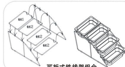
可拆式铁线架组合
