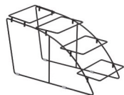
型号(规格) 尺寸(mm) MD035 520×275×315
